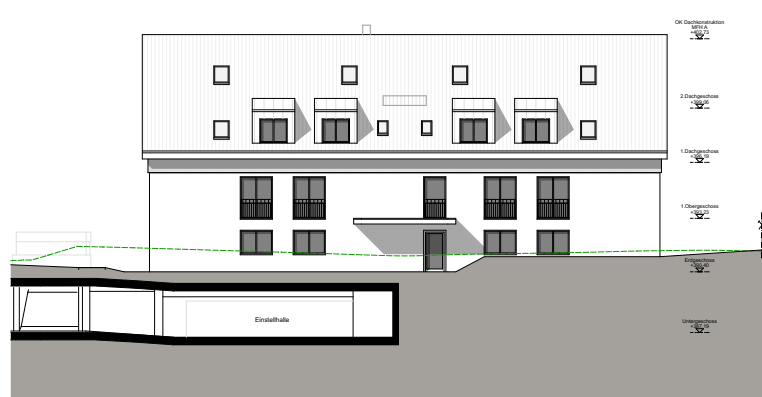
Haus A, Nordansicht
