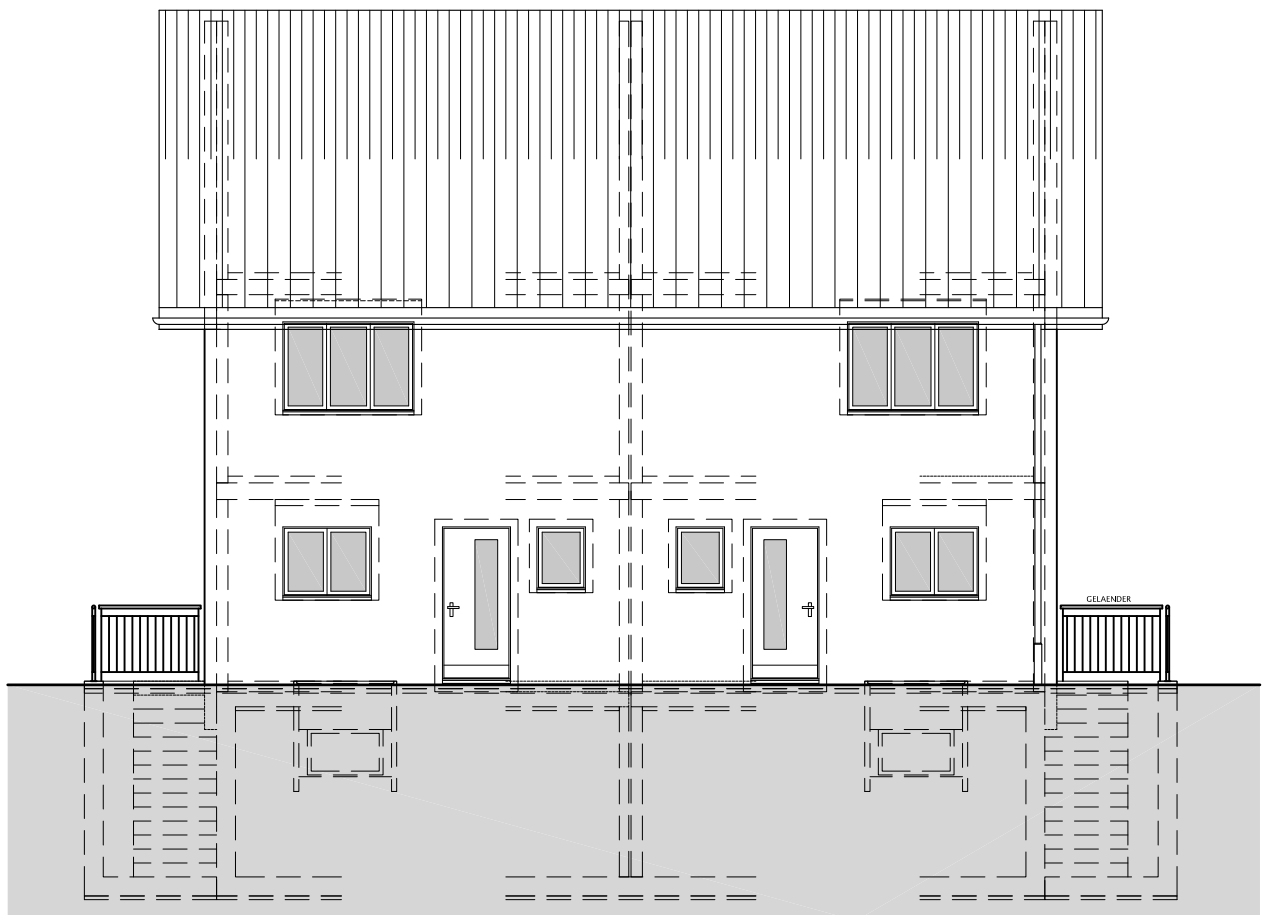
NORDFASSADE
