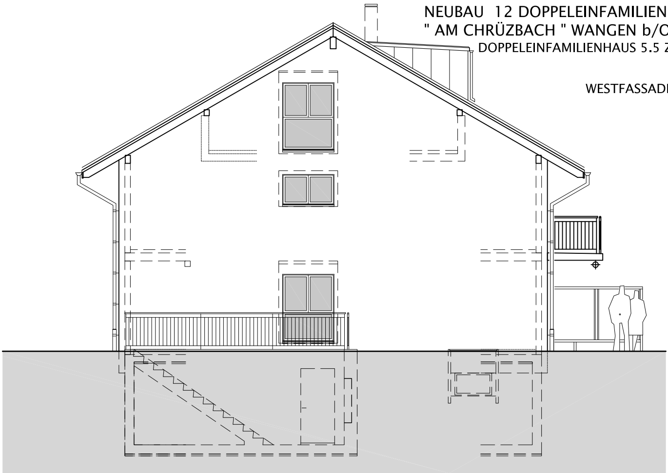
SÜDFASADE
