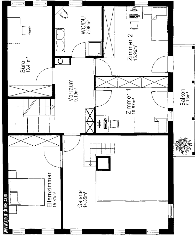
Obergeschoss
