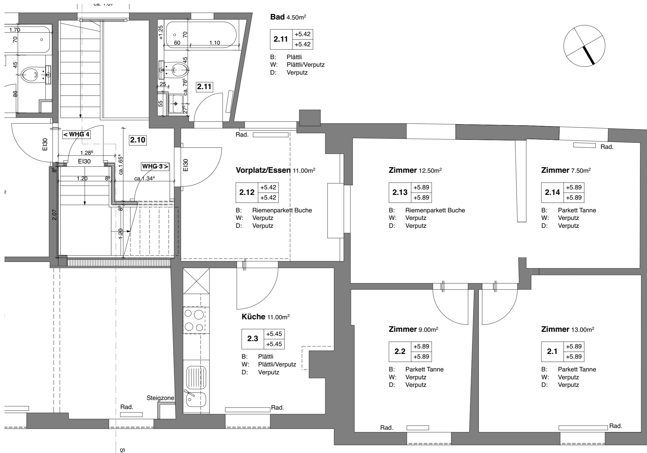
2. Obergeschoss
