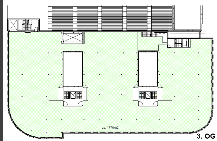
3. Obergeschoss
