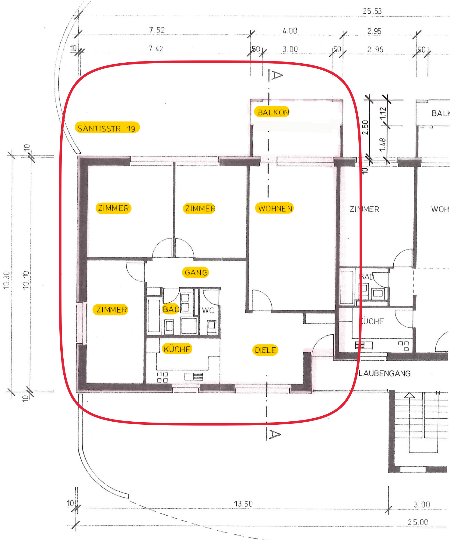
GRUNDRISS EG / 1.OG / 2.OG / 3.OG
