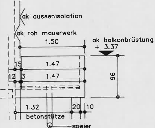
ansicht b, 1: 50
