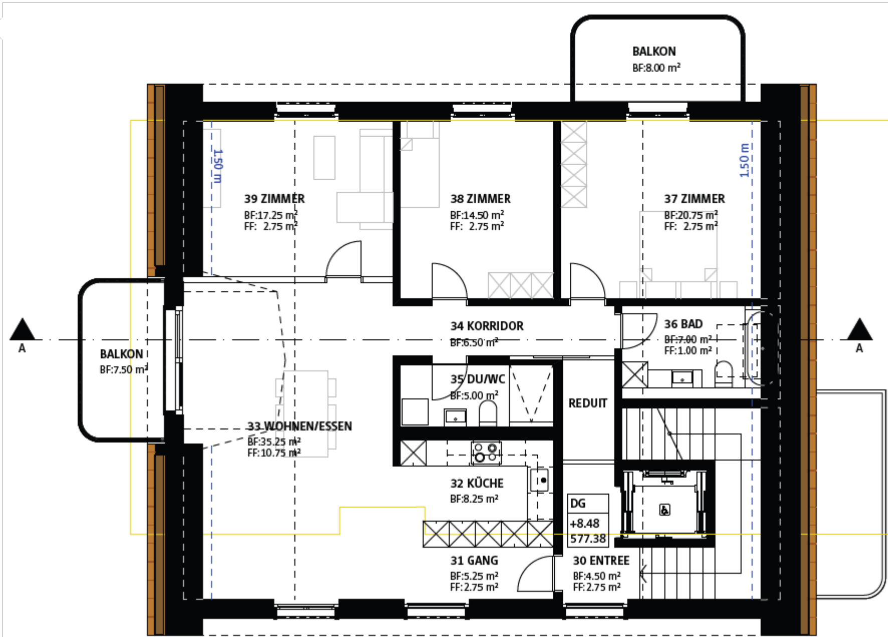
GRUNDRISS DACHGESCHOSS
