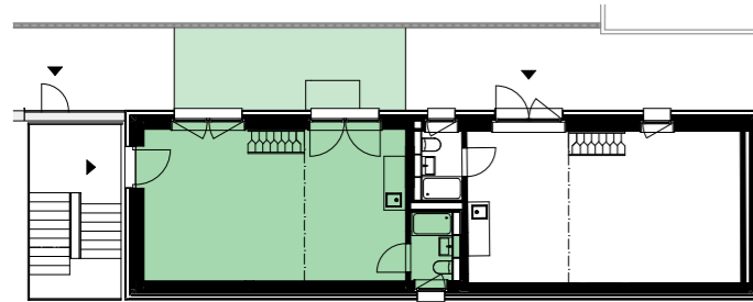
Erdgeschoss
