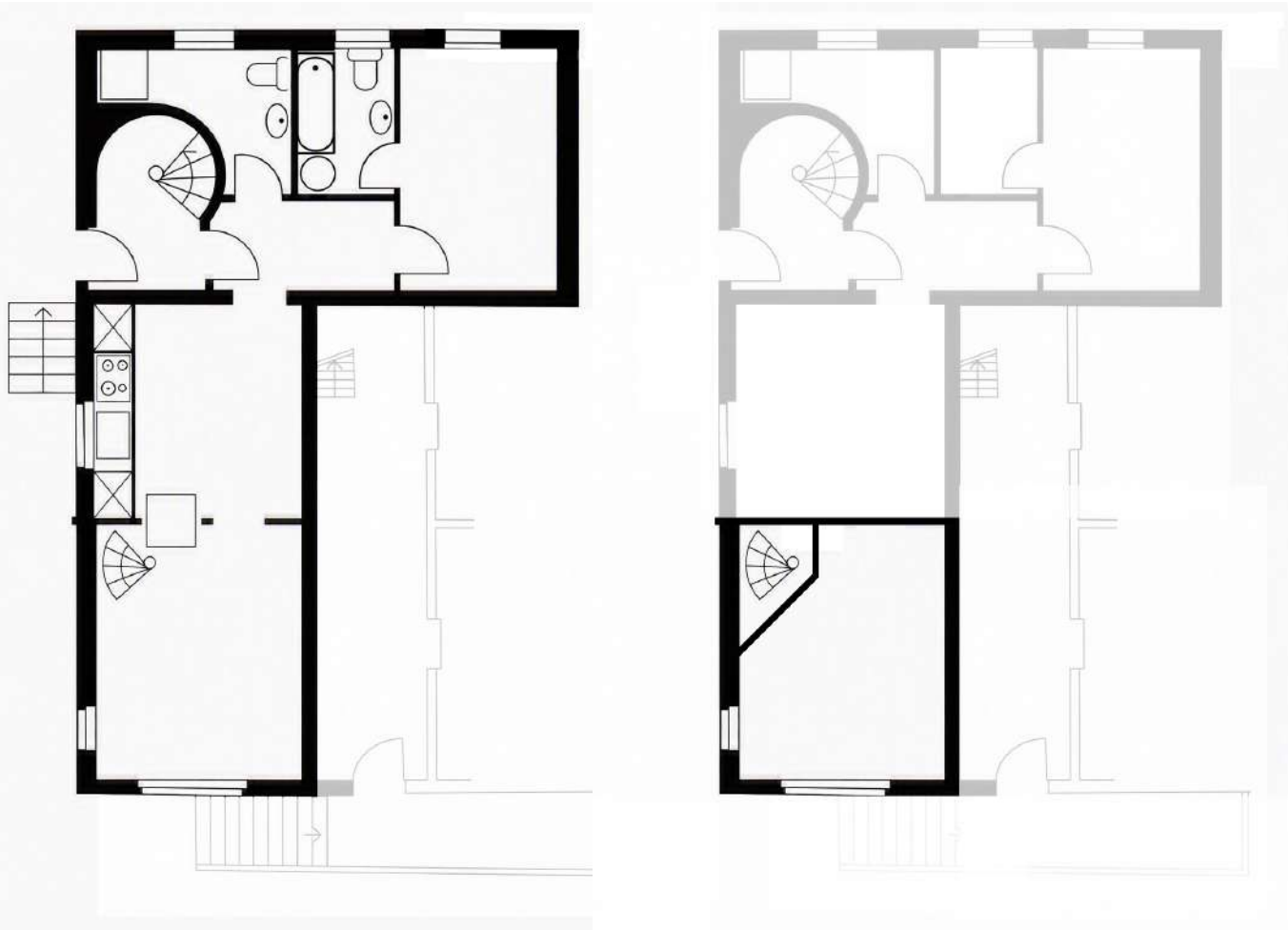
Obergeschoss Wohnung 1
