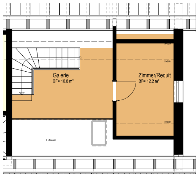
2.Dachgeschoss 23.0 m²
