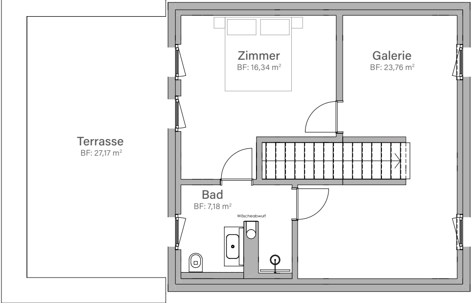
2. OG
