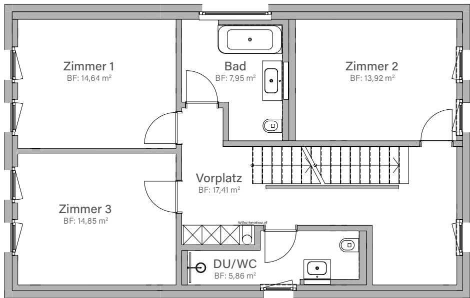
1. OG
