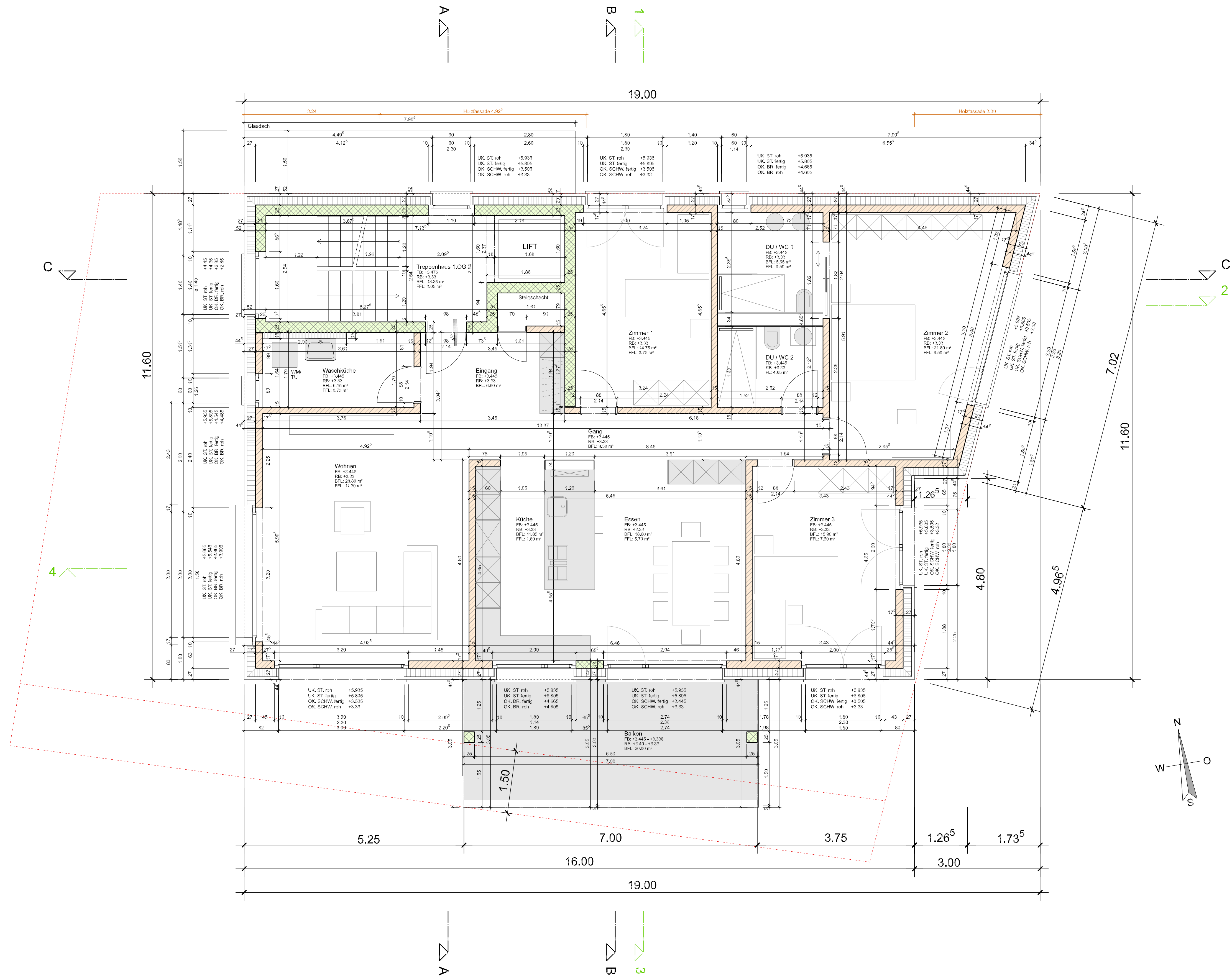
1. OBERGESCHOSS 1:50
