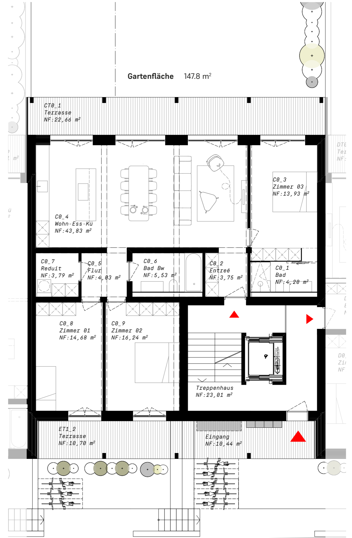
Grundriss EG
