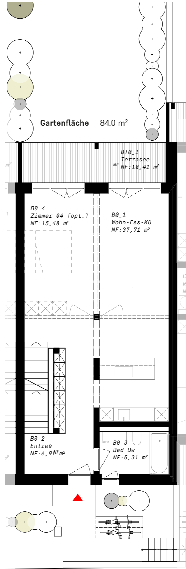
Grundriss EG
